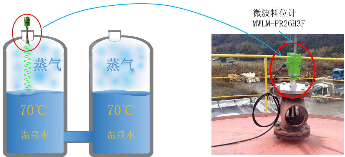
※图与照片：温泉水储槽设置微波料位计计测的樣子
